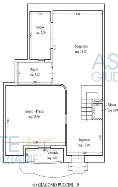
PIANTA PIANO TERRA h = 3,00 ml.
