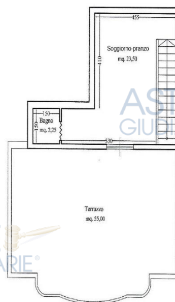
PIANTA PIANO SECONDO h = 2,40 ml.
